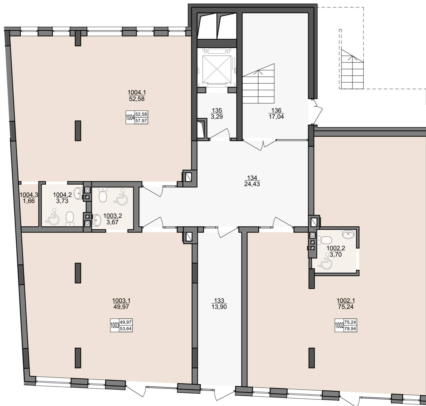
План першого поверху
